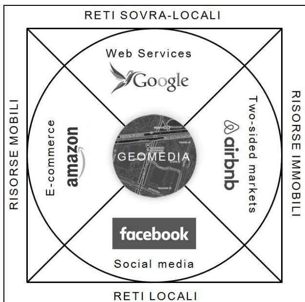
Fig. 1 - Il codespace .
